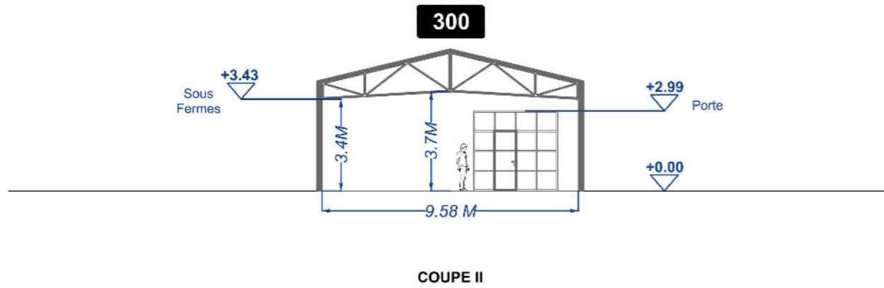
COUPE II
